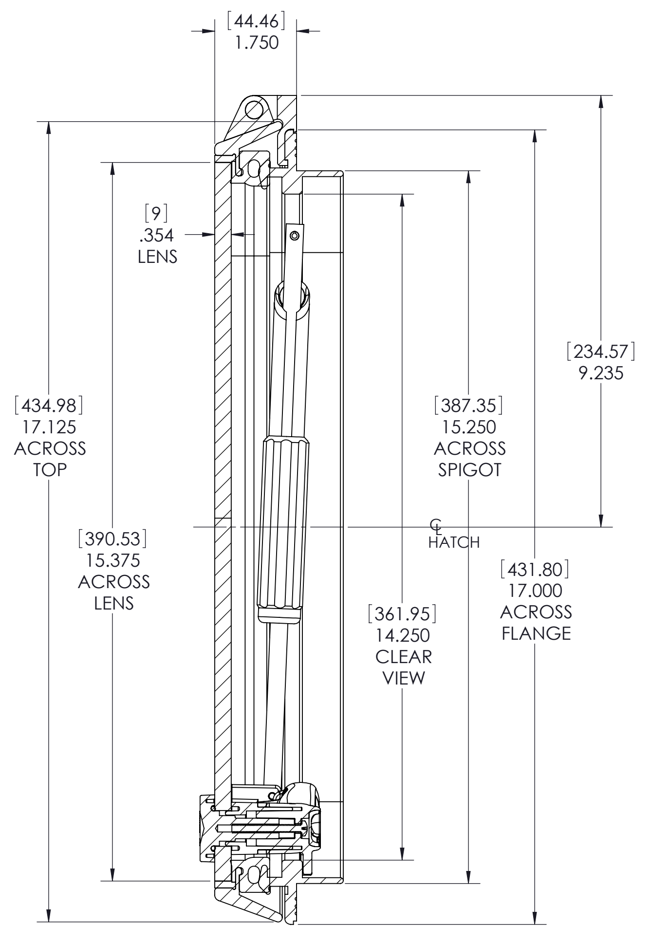
SECTION A-A
